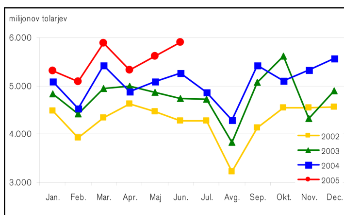
Slika 3.7.2. Izdatki obveznega zdravstvenega zavarovanja za zdravila v obdobju 2002–2004 in od januarja do junija 2005.
