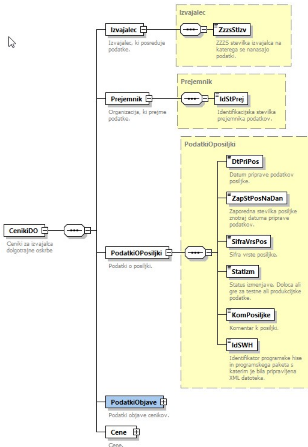
Slika 1: Krovna struktura datoteke
